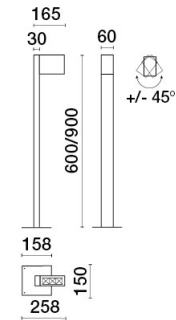
CON BASSETTA A PAVIMENTO WITH FLOOR PLATE
