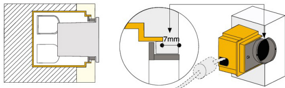
Scatola da immerare tipo 503E + adattatore in dotazione Wall box type 503E + adaptor included
