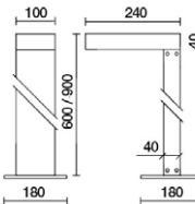
CON BASETTA A PAVIMENTO WITH FLOOR PLATE
