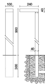
CON PALO DA INTERRARE WITH POLE TO BE BURIED
