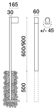
CON PALO DA INTERRARE POLE FOR IN-GROUND MOUNTING
